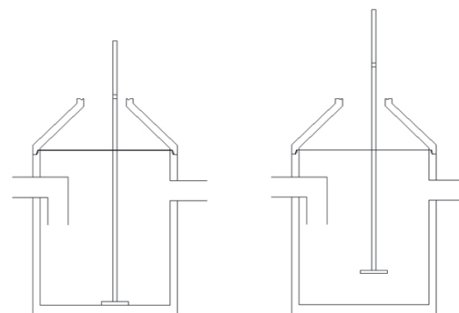
Figur 1 slammåling
